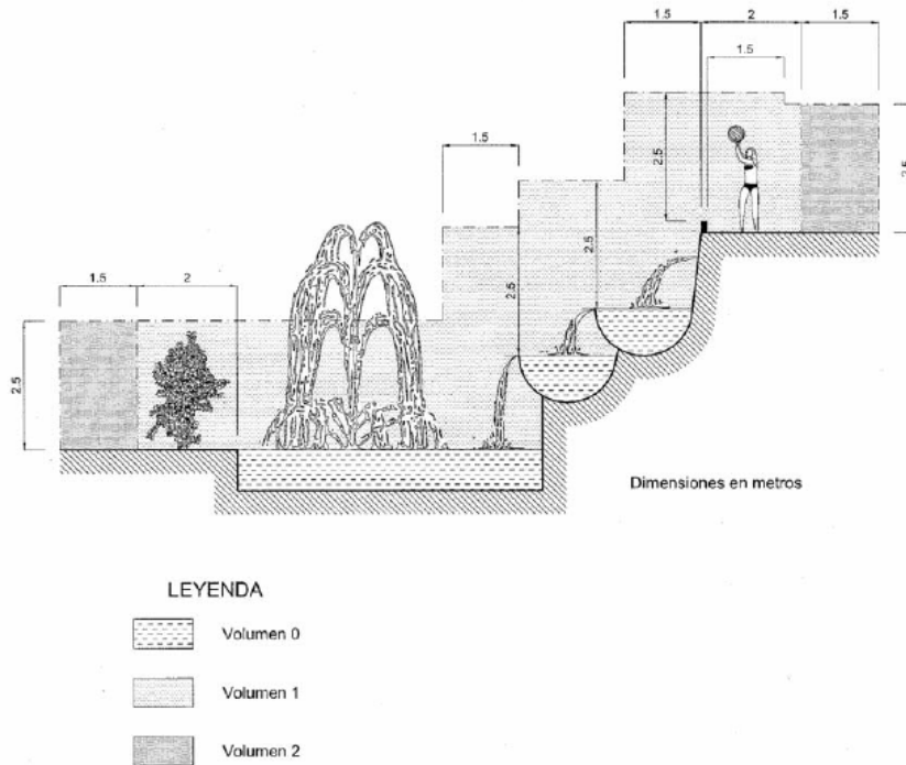
Figura 5. Volúmenes de protección en fuentes
