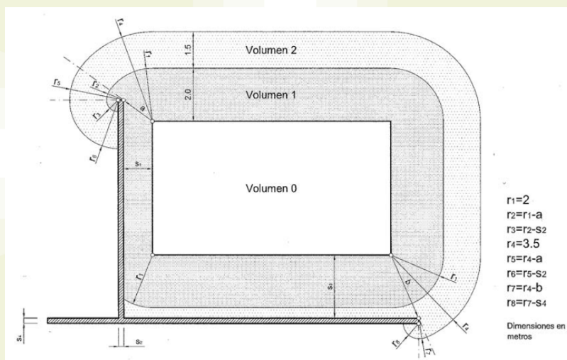
Figura 4. Volúmenes de protección en piscinas con paredes
