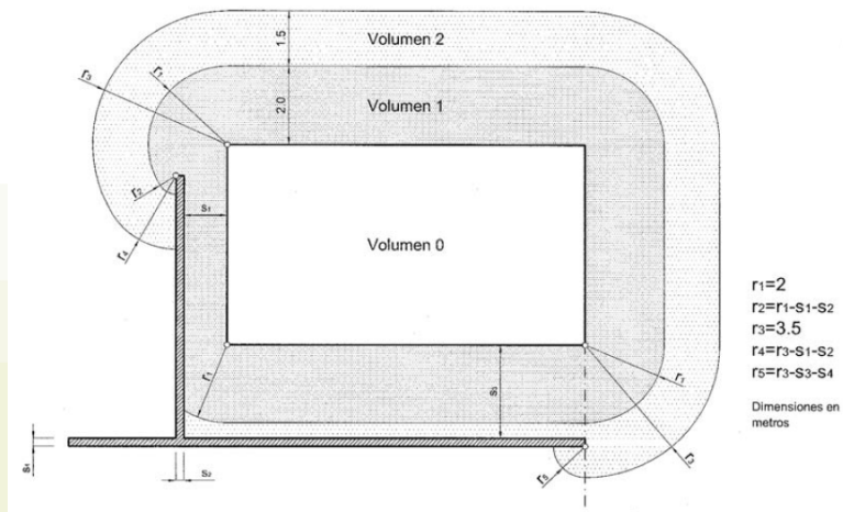
Figura 4. Volúmenes de protección en piscinas con paredes
